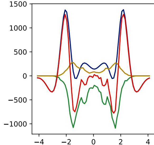
DOPE
