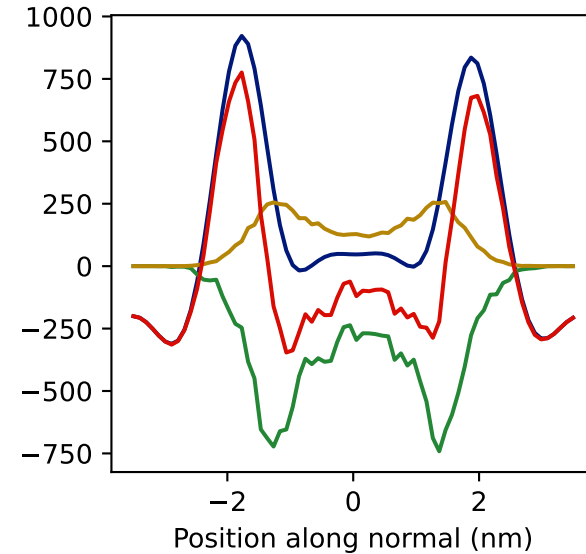
POPG
