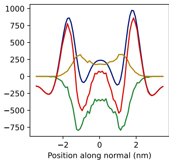
DMPG
