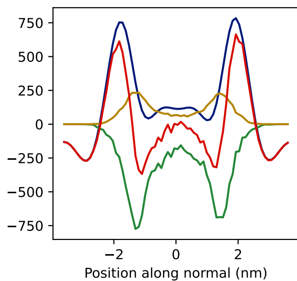
DOPG
