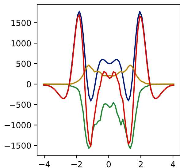
DMPE
