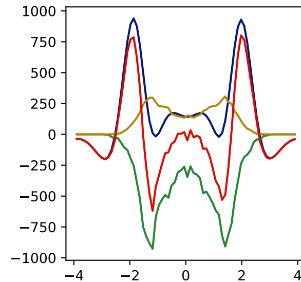
POPC
