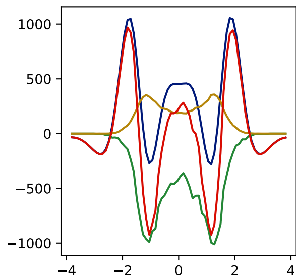
DMPC
