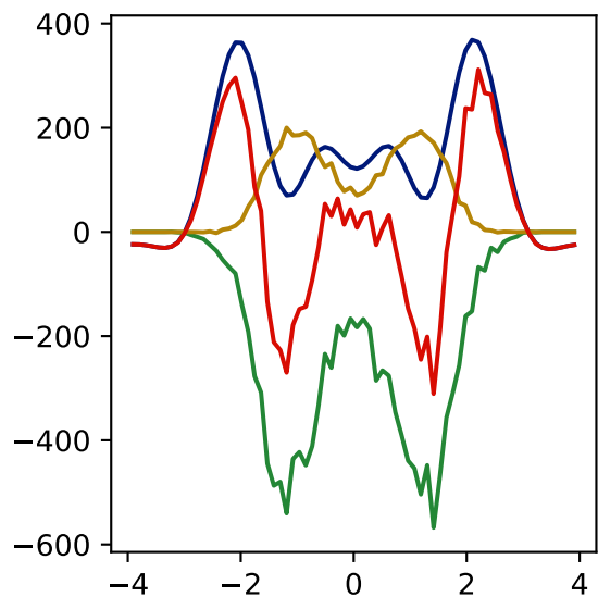
DPPE
