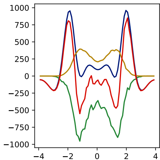
DPPC
