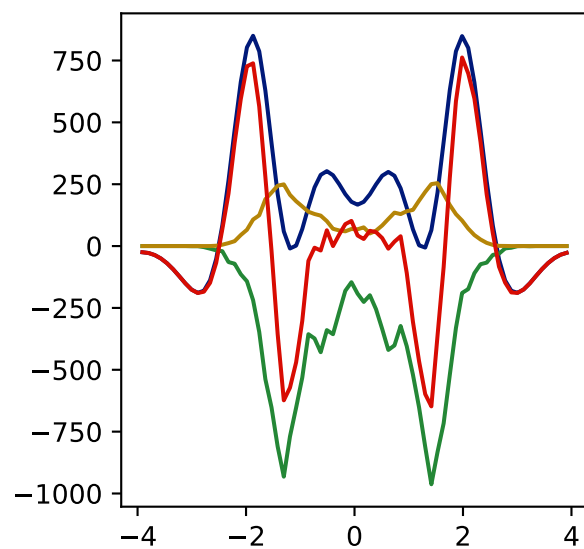
DOPC
