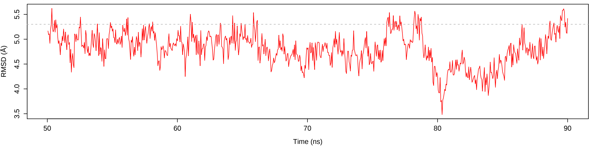
(D) Cis subunit (350K)
