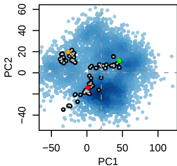
(D) GroEL ATP 7 (trans)
