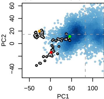
(E) GroEL E434K ATP 7 (cis)
