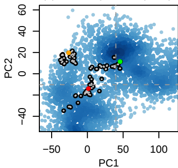
(F) GroEL E434K ATP 7 (trans)
