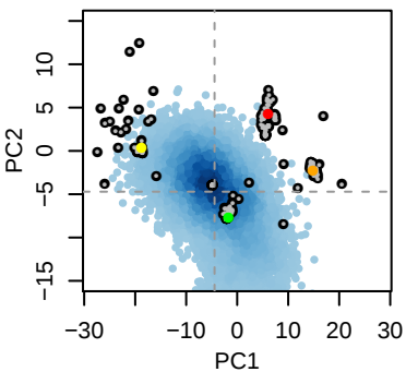
(E) GroEL E434K ATP 7 (cis)
