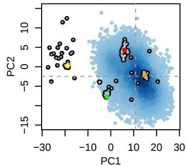
(D) GroEL ATP 7 (trans)
