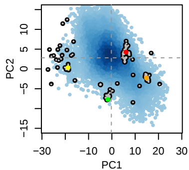
(F) GroEL E434K ATP 7 (trans)
