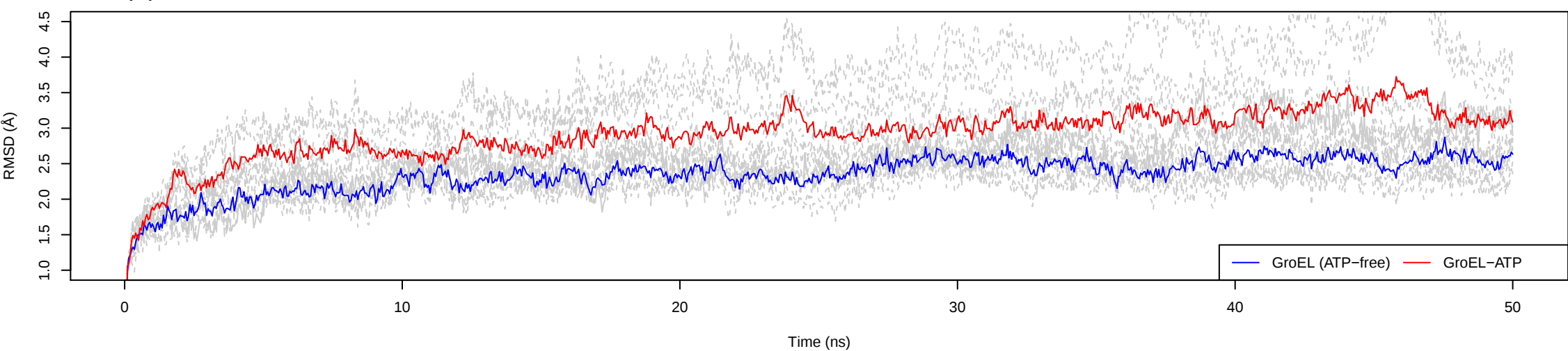
(B) Dimers
