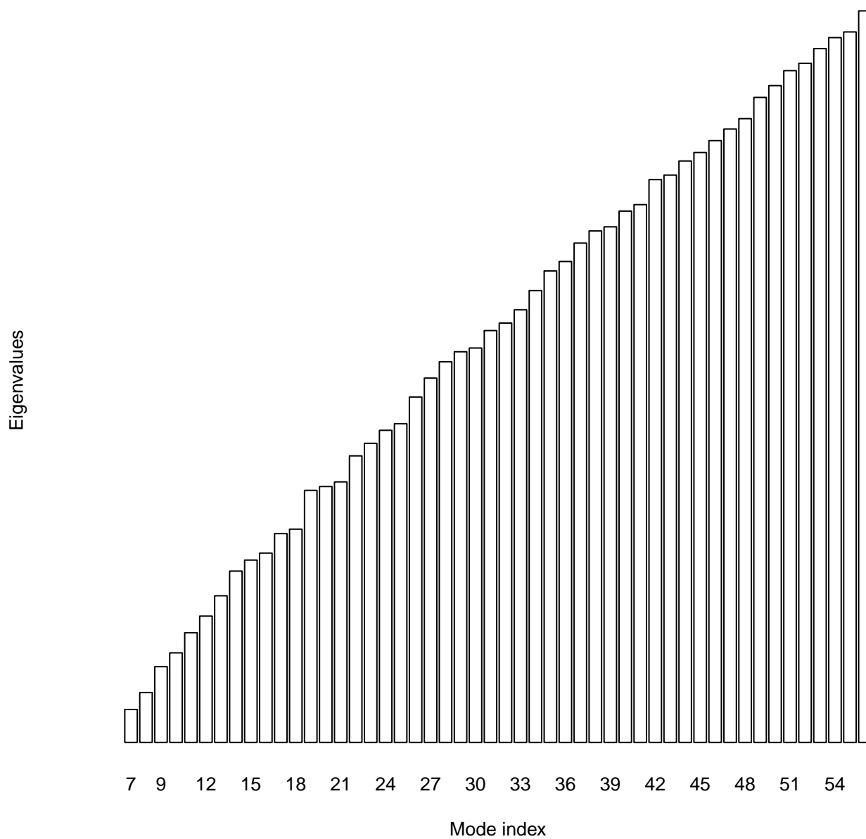
Eigenvalues plot for 1KKO.pdb
